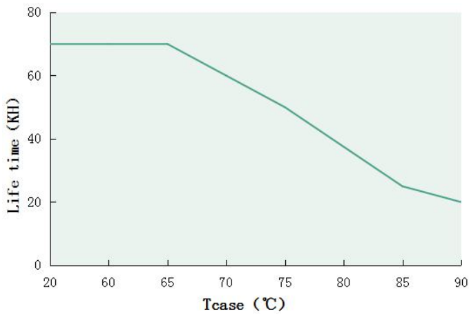
Tcase VS Lifetime(DL-100I-MAS)
