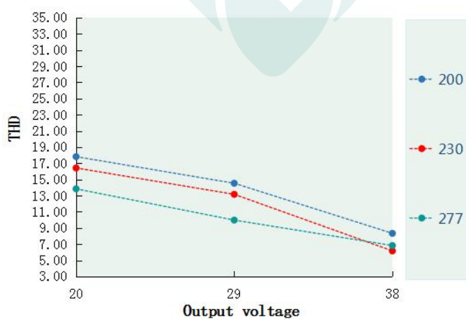
T.H.D. VS Output voltageDL-100I-V38P/A-MAS)
