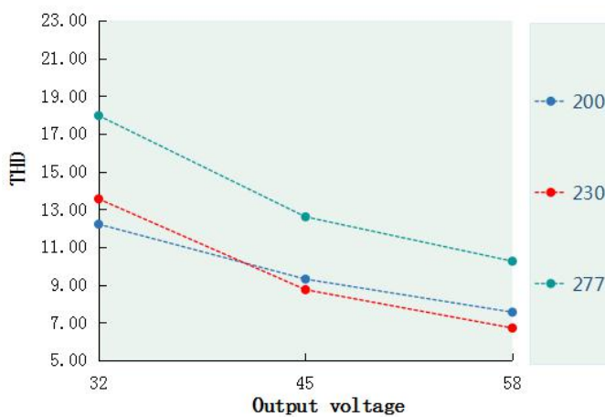
T.H.D. VS Output voltage(DL-100I-V58P/A-MAS)
