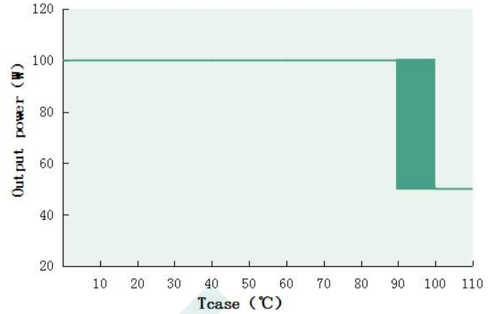
Output power VS Tcase (DL-100I-MAS)
