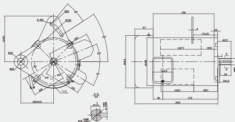
YCYGL8052外形图
