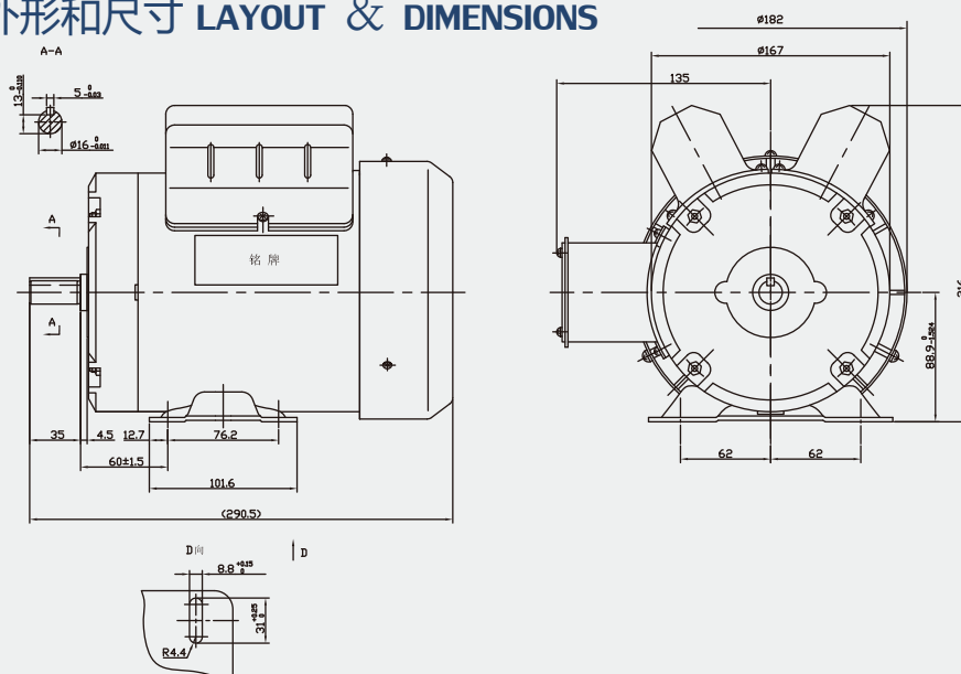
YCYN5652D-1外形图
