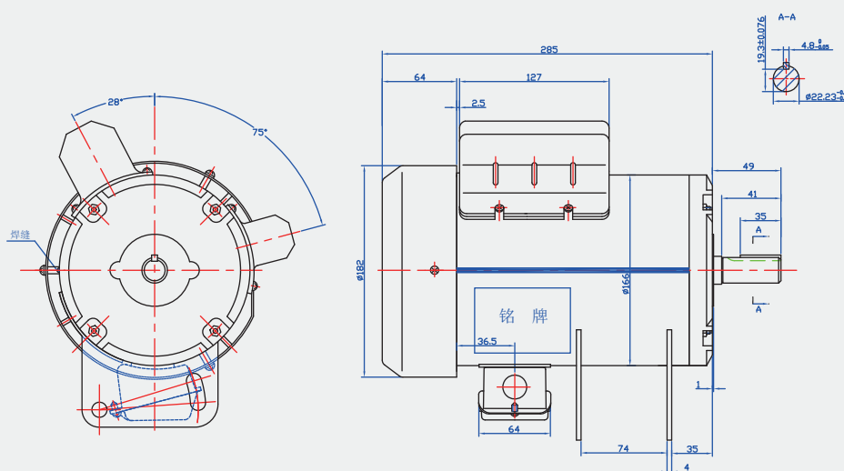
YCYN5692D-3外形图
