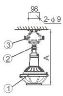
吸顶式(x) Ceiling type(x)
