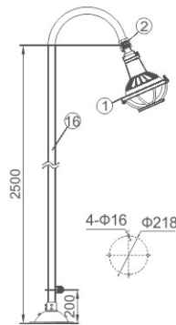
法兰式(f)/Flange type(f)
