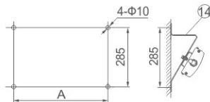
壁式/Wall type(b)
